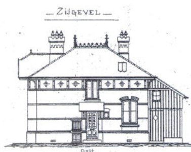
Tekening oostgevel, 1896 (bron: kopie tekening collectie bewoner)
